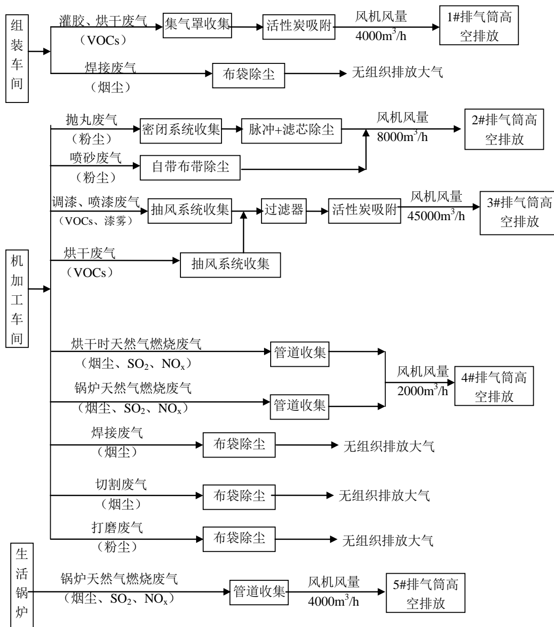
图 11 项目废气处理示意图
