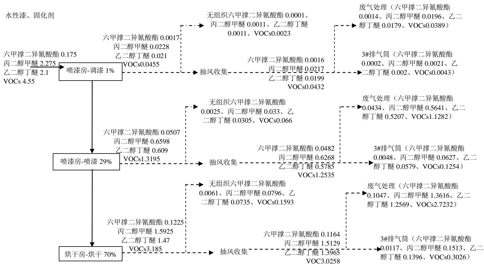
图 10 本项目喷漆工序 VOCs 平衡图（单位：t/a）
